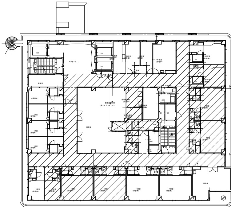
4階 平面図 (A3 S=1/300)
