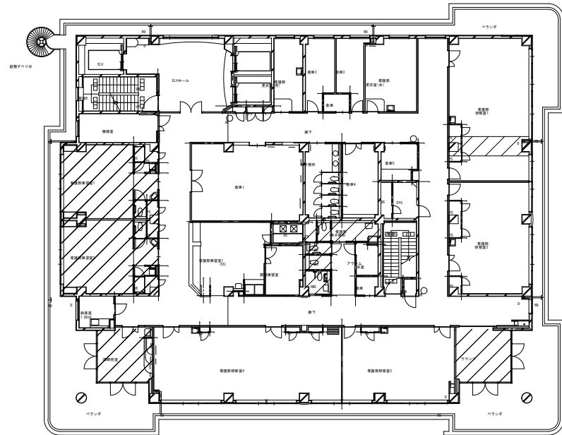
6階 平面図 (A3 S=1/300)
